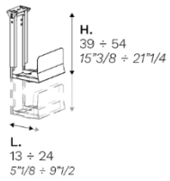
18. vasca di cablaggio regolabile in altezza
